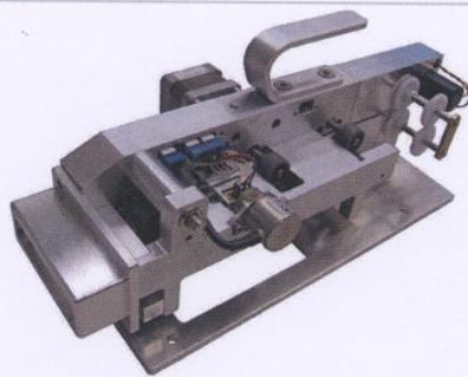
Entwerter-Einheit Validator
