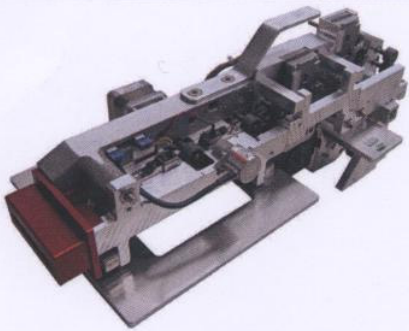
Ausgabe-Einheit Dispenser
